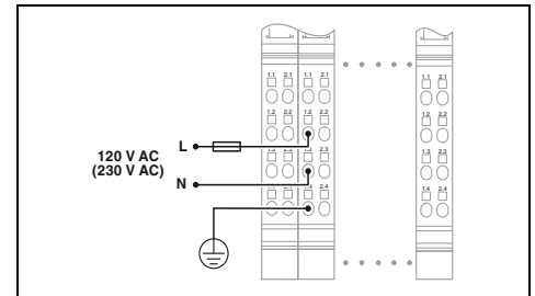
Питание 230 В перем. тона U_L , выборочно с предохранителем и диагностическим индикатором
