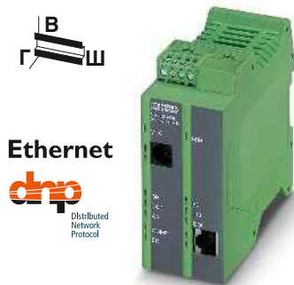
Модем для коммутируемых линий с разъемом для подключения к сети Ethernet (LAN)
