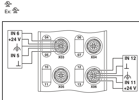
16 дискретных входов
