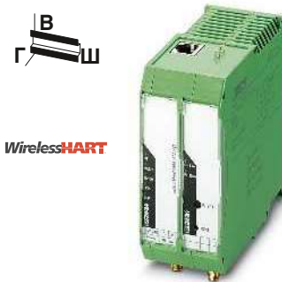
Шлюз WirelessHART, для использования по всему миру
