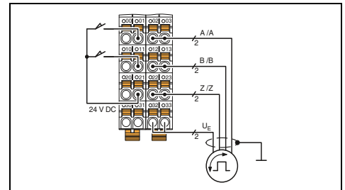
2 входа для счетчика, 2 интерфейса для инкрементального энкодера
