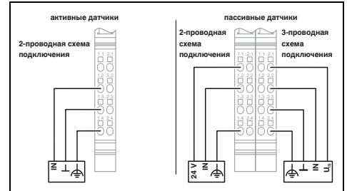
8 входов, с питанием датчика иницирующих сигналов
