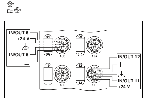
16 свободно настраиваемых входов или выходов
