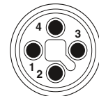
Расположение контактов штекера M12, 4 полюса, с механическим ключом типа T, вид со стороны штыревой части
