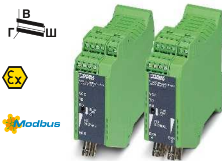
RS-485-2-проводной PCF-волокно и стекловолоконно (многомодовое)
