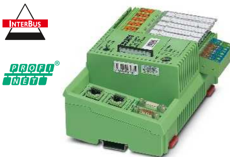
Высокопроизводительный, с интерфейсом ведомого устройства INTERBUS
